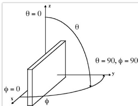
Polar Coordinates
