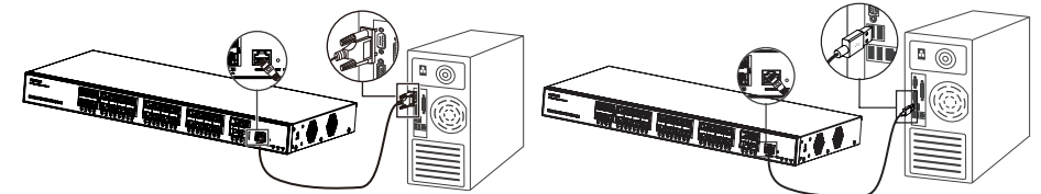
Anbindung über den Konsole-Port (USB)
