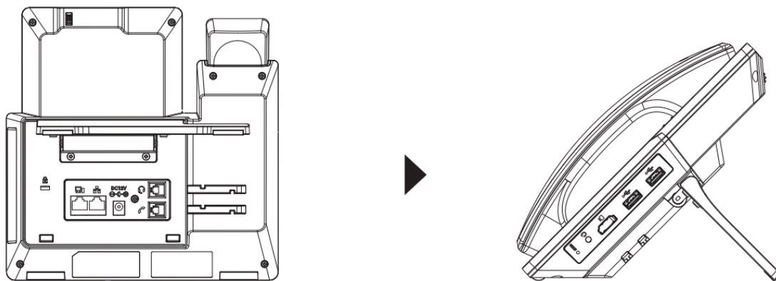
GXV3470 Phone Stand
