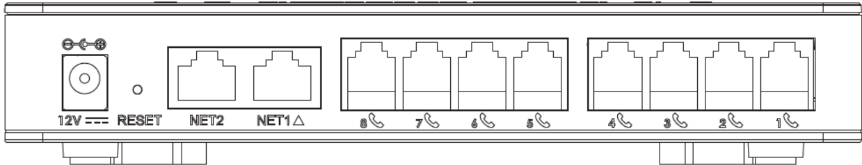
HT818 V2 Ports
